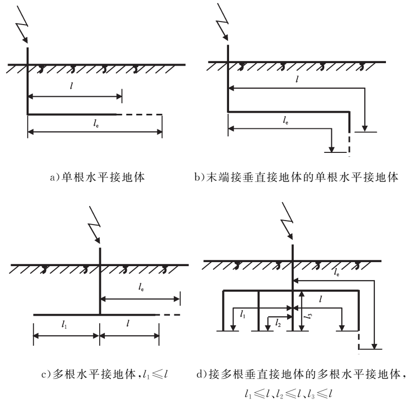
图 D.2 接地体有效长度的计量
