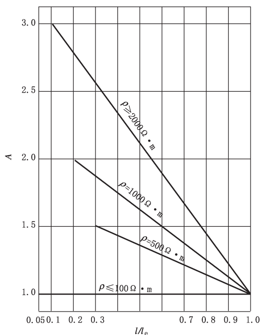
图 D.1 换算系数 A
